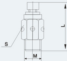
■ 外观图/overall Dimension
