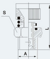
■ 外观图/overall Dimension
